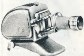
Noris-Trumpf S 1 projektiionsapparat 5x5 med Katagon 1:2,8/85 mm, til 150 watt's lampe; asphærisk kondensersystem, med vekselslæde; incl. lampe . 225,00 Consten stativ-model III . 228,00
