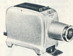
AGFA OPTICUS »100« 5x5 projektionsapparat med Agomar 1:3,5/85 mm, 220 v/100 w lampe, asphærisk kondensatorsystem, vekselskakt og automatisk tilpasning
